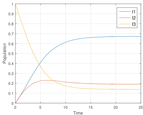
(d) ODE Model; D = 0.05
